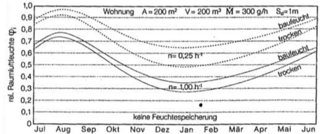
Bild 9: Jahresverlauf der Raumlufffeuchte bei baufeuchten und im hygrischen Gleichgewicht stehenden Bauteilen bei zwei Luftwechselraten
