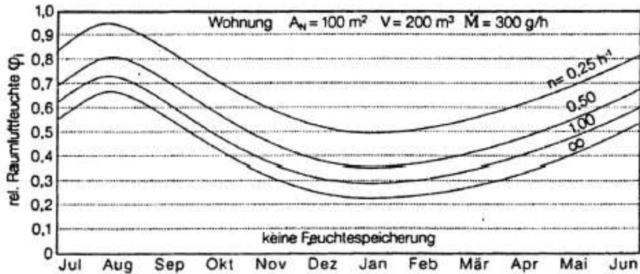
Bild 7: Jahresverläufe der Raumlufffeuchte bei verschiedenen Luftwechselraten
