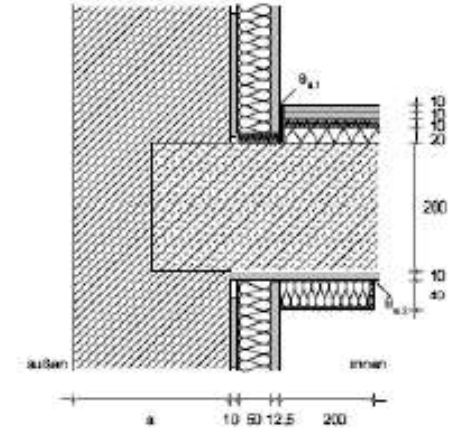
Sanierungsvariante D-1b, Verbundplatte
