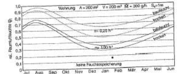
Bild 9: Jahresverlauf der Raumluftfeuchte bei beaufeuchteten und im hygrischen Gleichgewicht stehenden Bauteilen bei zwei Luftwechselraten
