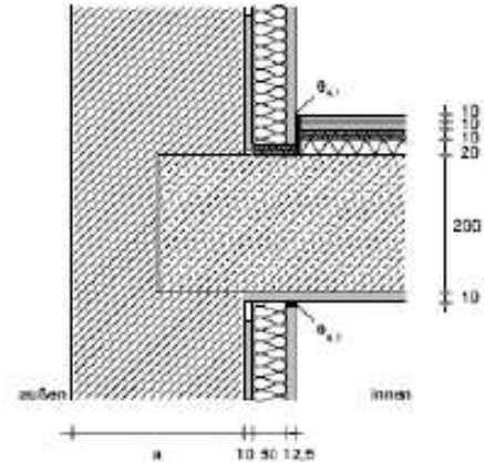
Sanierungsvariante D-1a, Verbundplatte
